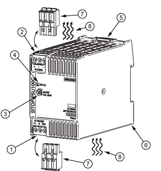
Bild 2: Aufbau Figure 2: Design Figura 2: Diseño 图 2: 结构 Figure 2: Structure Figura 2: Struttura Рисунок 2: Конструкция Resim 2: Yapı
